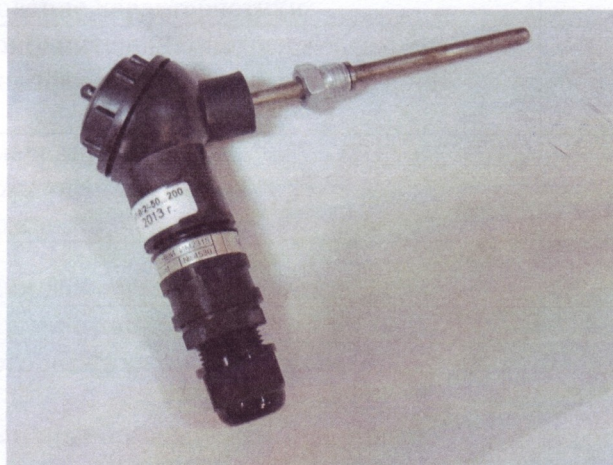
Рисунок 2 - Преобразователь в сборе с термопреобразователем сопротивления Пломбирование преобразователей измерительных ИМ2315 не предусмотрено.
